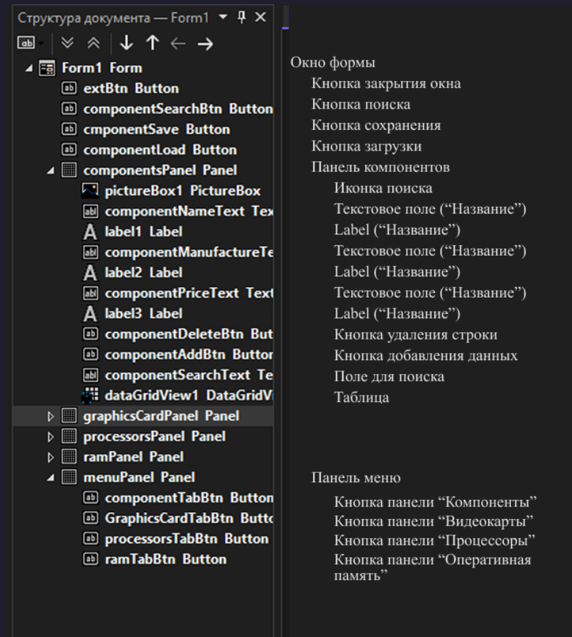
Рисунок 4.9 – Структура формы
